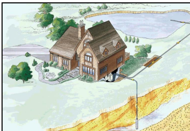
Εικόνα 5: Μικτό ανοικτό σύστημα αβαθούς γεωθερμίας
