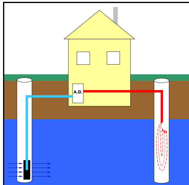
Εικόνα 4: Ανοικτό σύστημα αβαθούς γεωθερμίας μονού φρέατος
