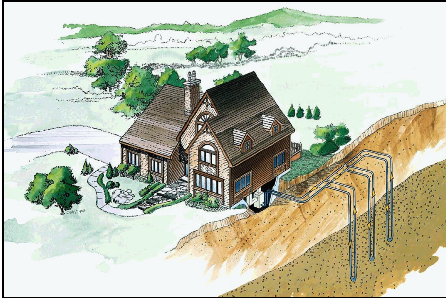
Εικόνα 13: Κατακόρυφο σύστημα αβαθούς γεωθερμίας με παράλληλο γεωεναλλάκτη
